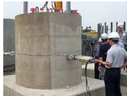
3. Splitteren deler opp fjellet/betongen med 400 tonn's kraft.
